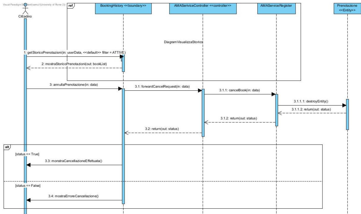
Figura 32: Sequence Diagram — Annullare prenotazione
