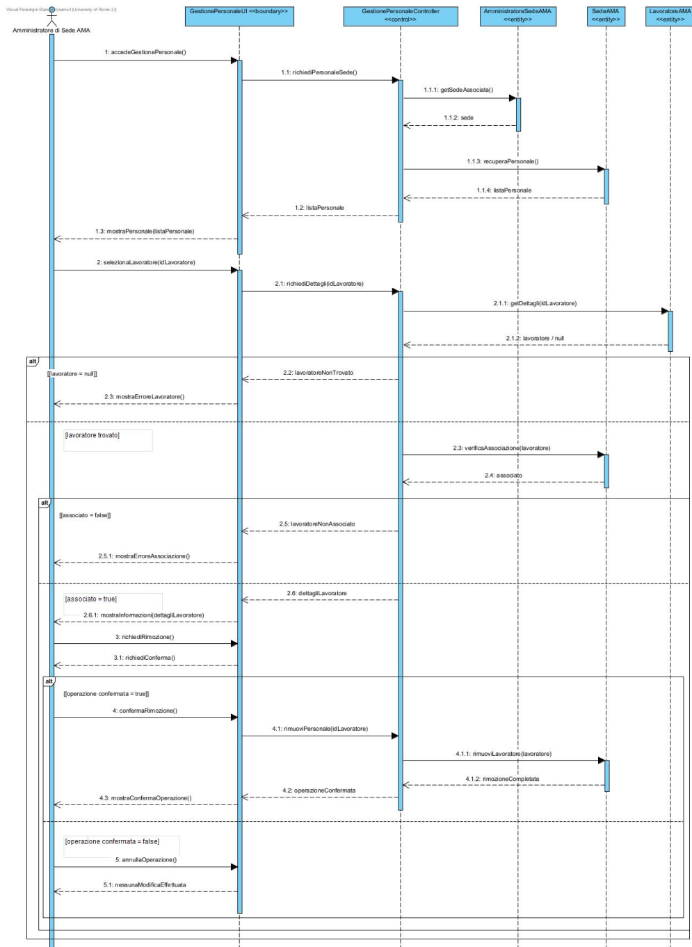
Figura 46: Sequence Diagram — Rimuovere personale
