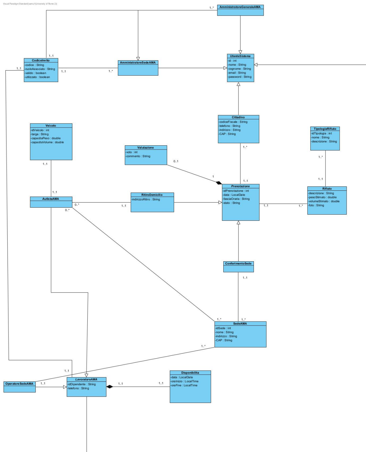
Figura 49: Class Diagram — Versione Unrefined (Modello di Dominio)
