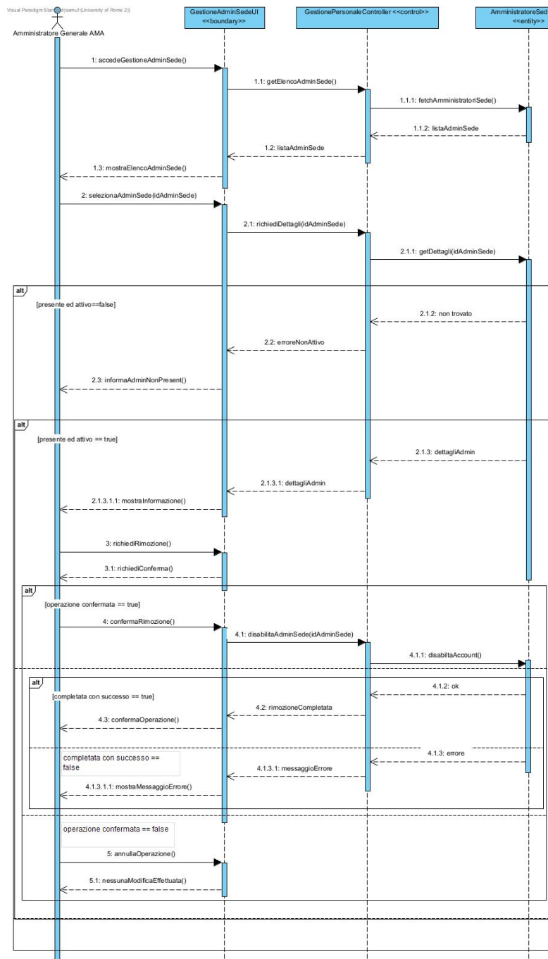
Figura 48: Sequence Diagram — Rimuovere amministratore di sede AMA
