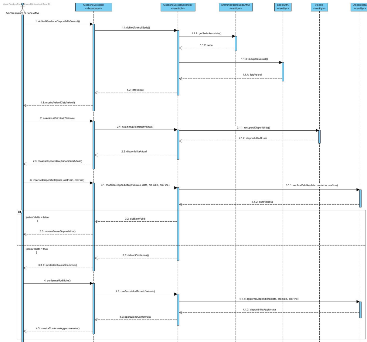
Figura 43: Sequence Diagram — Gestire disponibilità dei veicoli
