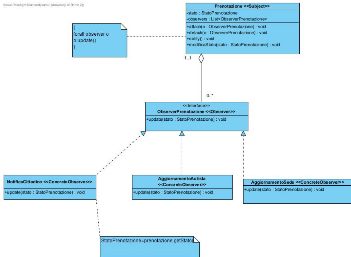
Figura 51: Struttura UML del Design Pattern Observer applicato a MyAma
